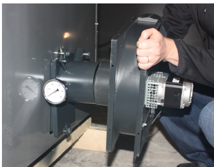
Asenna savukaasuimuri kiinni adapteriin (savuputki). Tiivistykseen voi käyttää lämmönkestävää massaa tai tiivistenarua.
