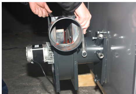
Kiristä imurin lukituspultti ja asenna savusolan jatkoputki.
