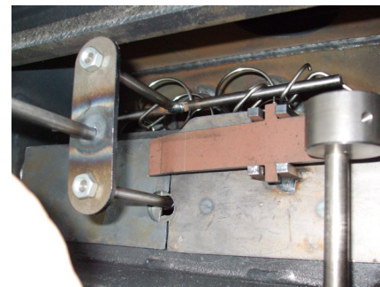
9. Asenna konvektiokanavan kannet ja keinuvipu paikoilleen.
