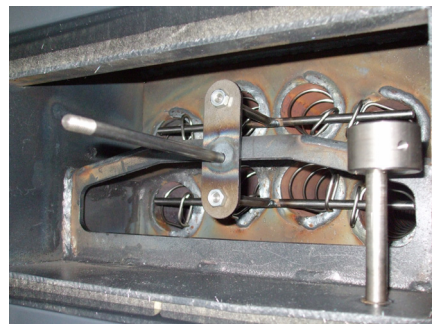
8. Asenna kaikki spiraalit ja nostotanko paikoilleen kuvan osoittamalla tavalla.
