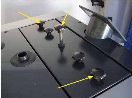
1. Avaa ulommat ja keskimmäinen tähtinuppi ja nosta puhdistusluukku pois.
